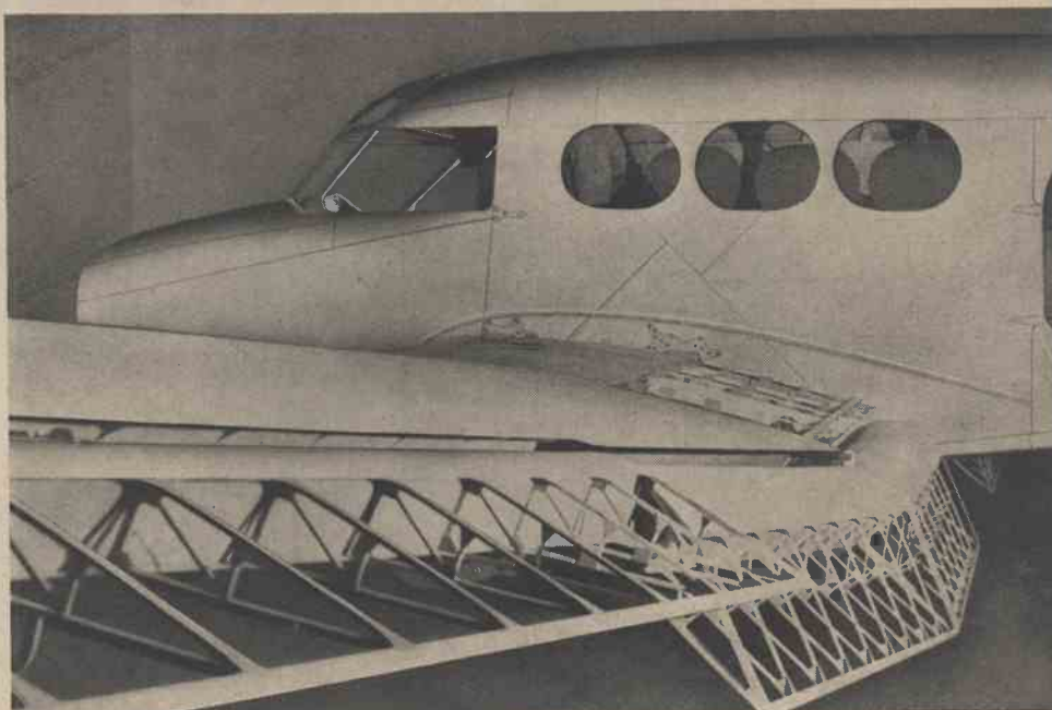
Kabinen med venstre Vinge, med Balanceklapper og „Flaps“
